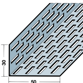
Profitec 9071 ventilationsprofil.
