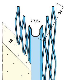
Profitec 1005 pudseprofil.
