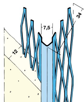
Profitec 1007 pudseprofil.
