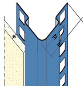
Profitec 30 108 Hjørneprofil.
