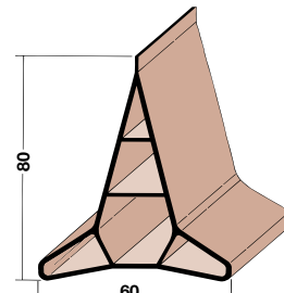
Profitec 3908 fugeprofil.
