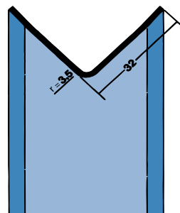
Profitec 2041 kantbeskyttelsesprofil.
